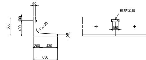
構造図
