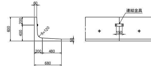
構造図
