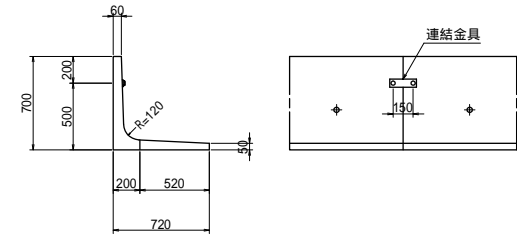
構造図
