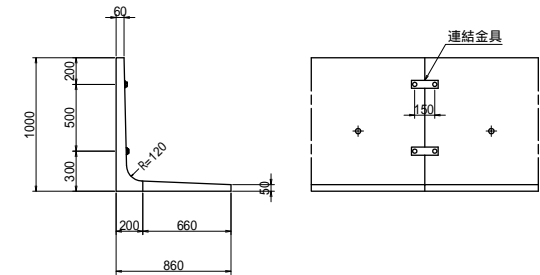
構造図
