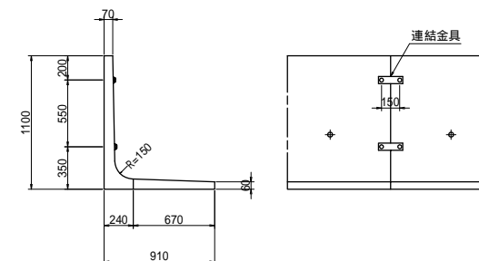
構造図
