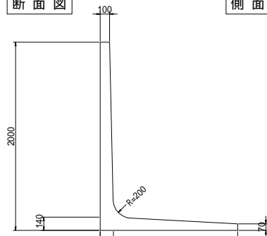
断面図
