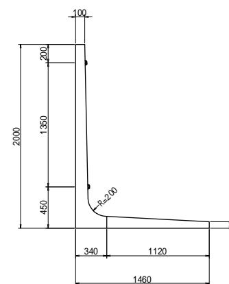
構造図
