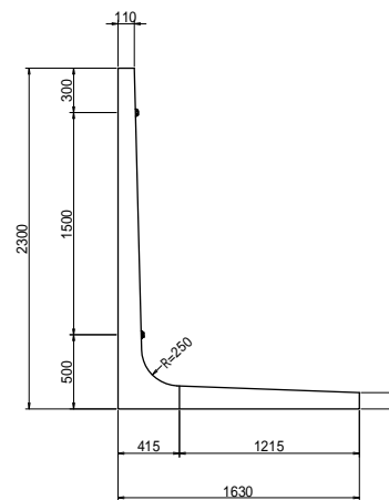
構造図
